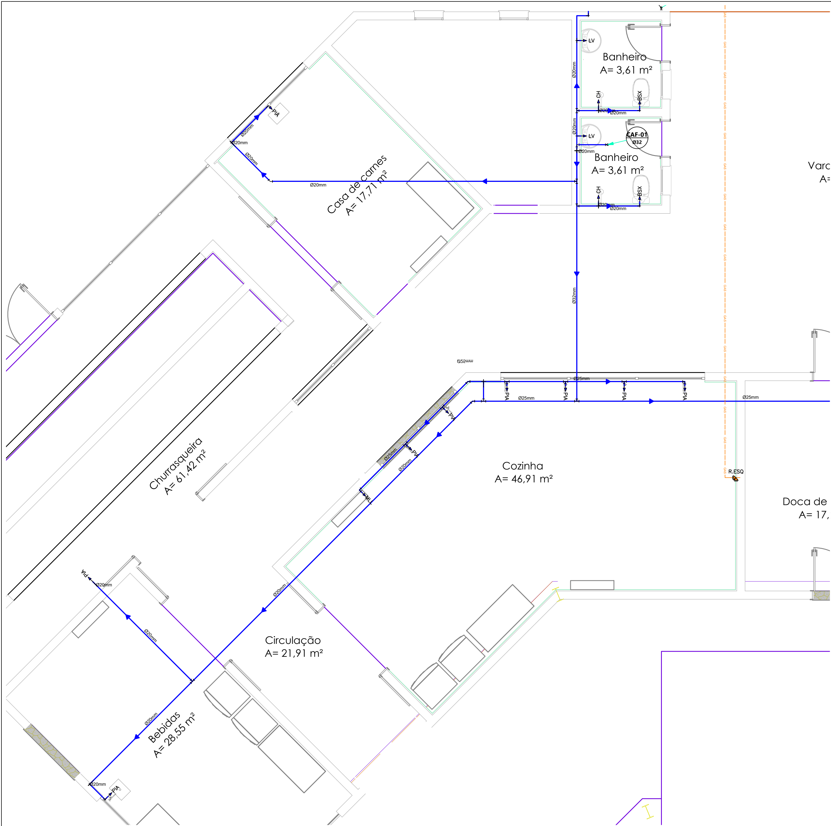
Projeto água fria - Trecho 1 Trecho 1 - Escala 1/50
