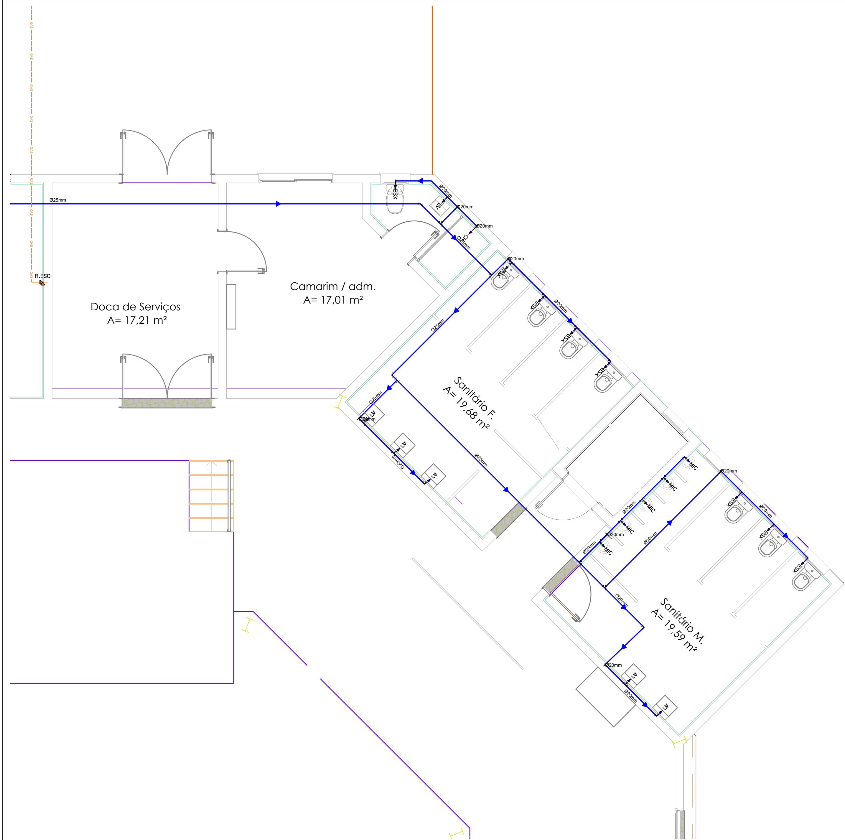
Projeto água fria Trecho 2 - Escala 1/50
