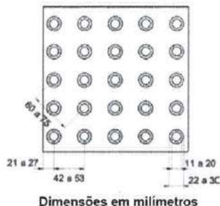
Dimensões em milímetros Sinalização tátil de alerta – Modulação do piso
