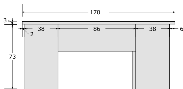
VISTA C
