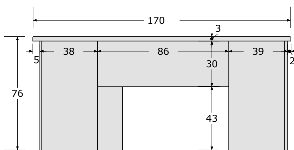
VISTA B
