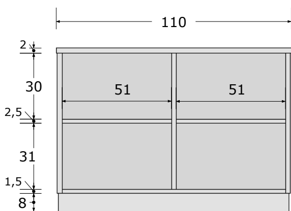
VISTA INTERNA
