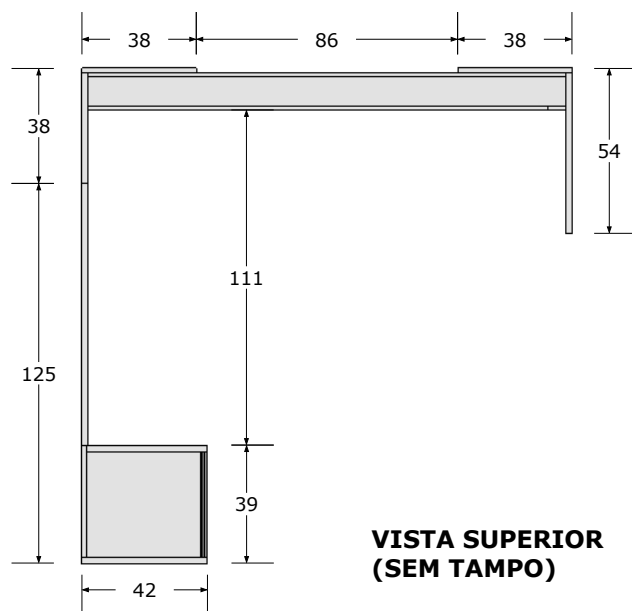
VISTA SUPERIOR
