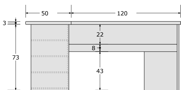
VISTA A
