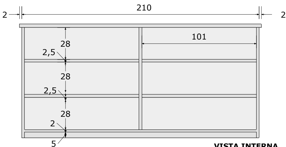
VISTA INTERNA
