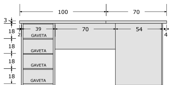
VISTA D
