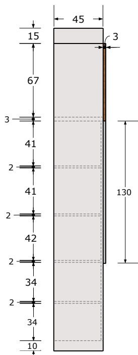
VISTA LATERAL
