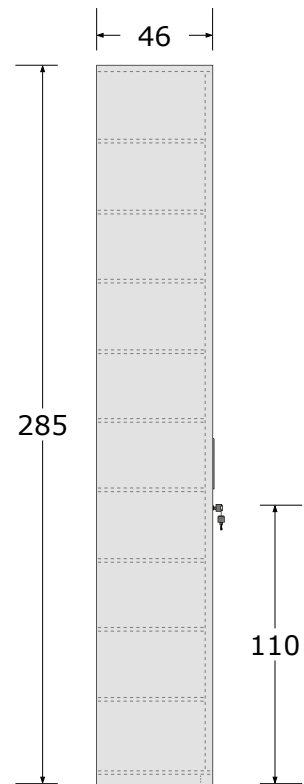
VISTA LATERAL
