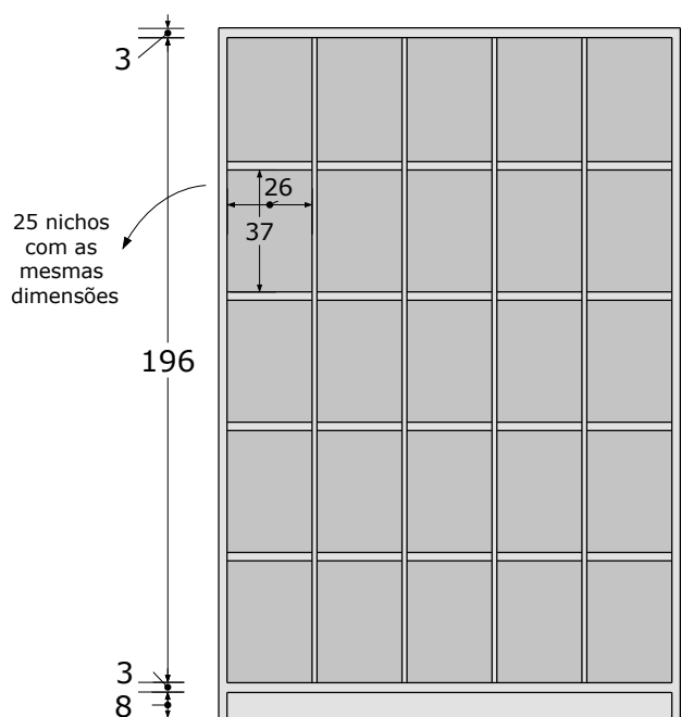
VISTA INTERNA
