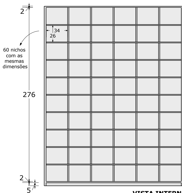
VISTA INTERNA
