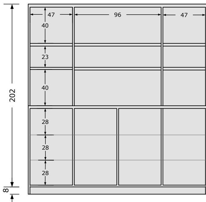
VISTA INTERNA
