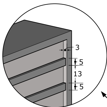
VISTA AA
