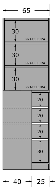
VISTA BB
