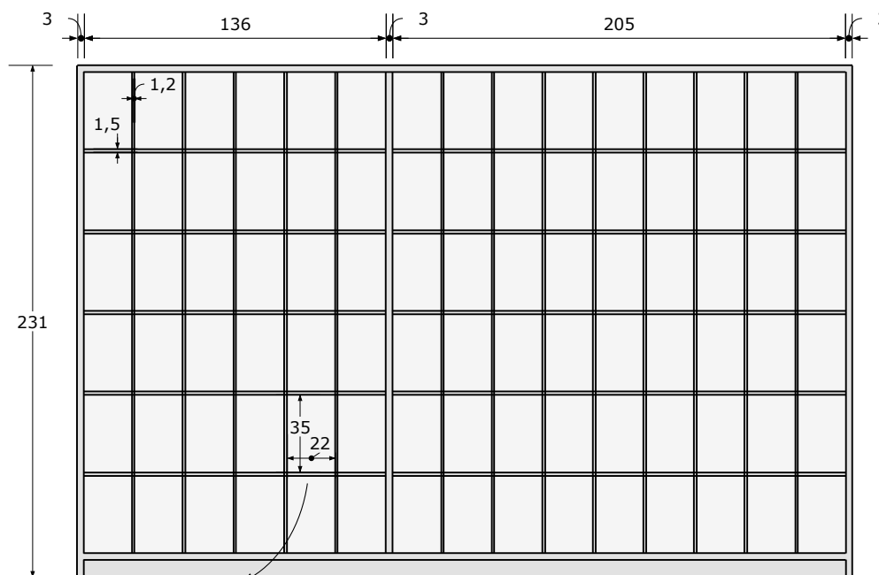
VISTA INTERNA
