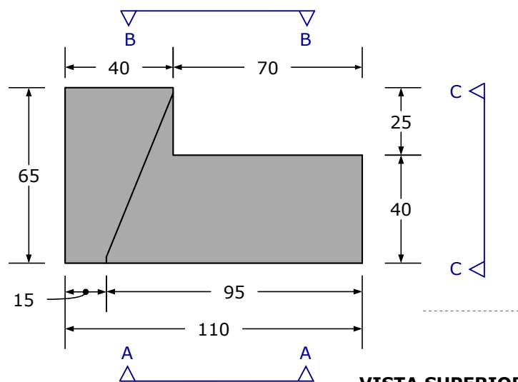
VISTA SUPERIOR
