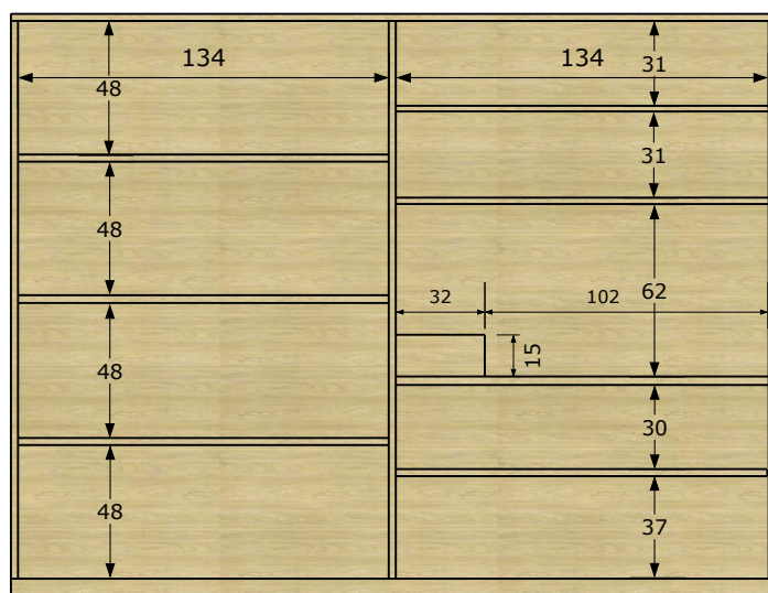
VISTA INTERNA
