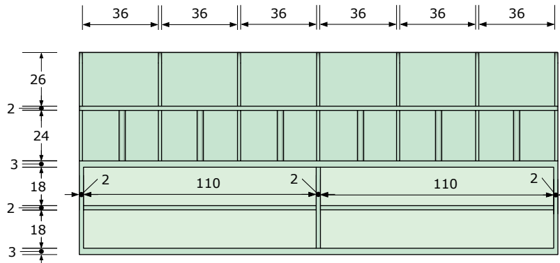
VISTA FRONTAL INTERNA
