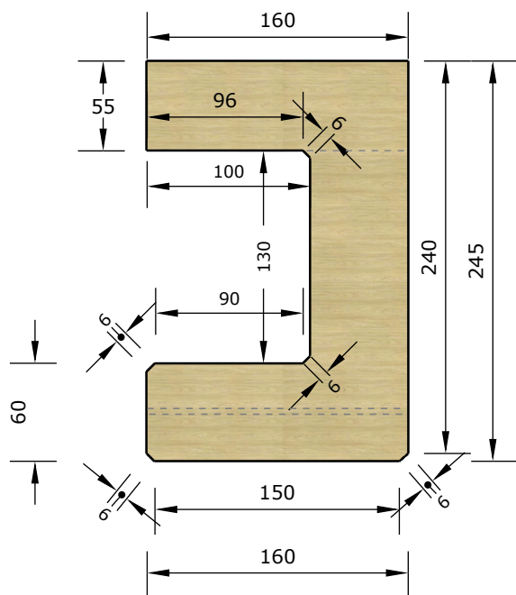
VISTA SUPERIOR
