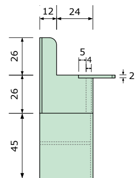
VISTA LATERAL INTERNA
