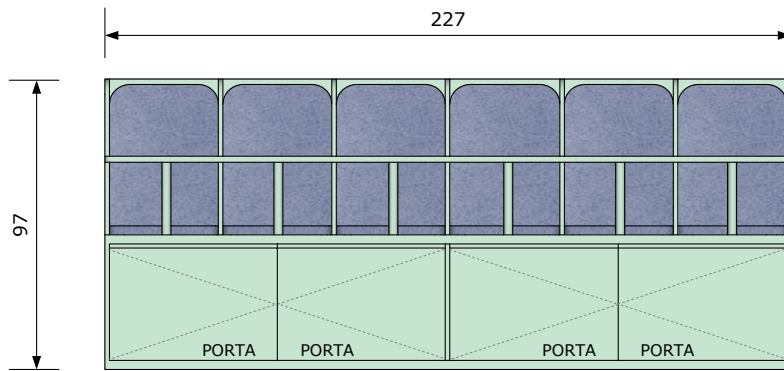
VISTA FRONTAL (com almofadas)
