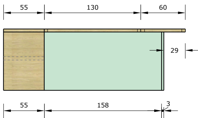
VISTA LATERAL
