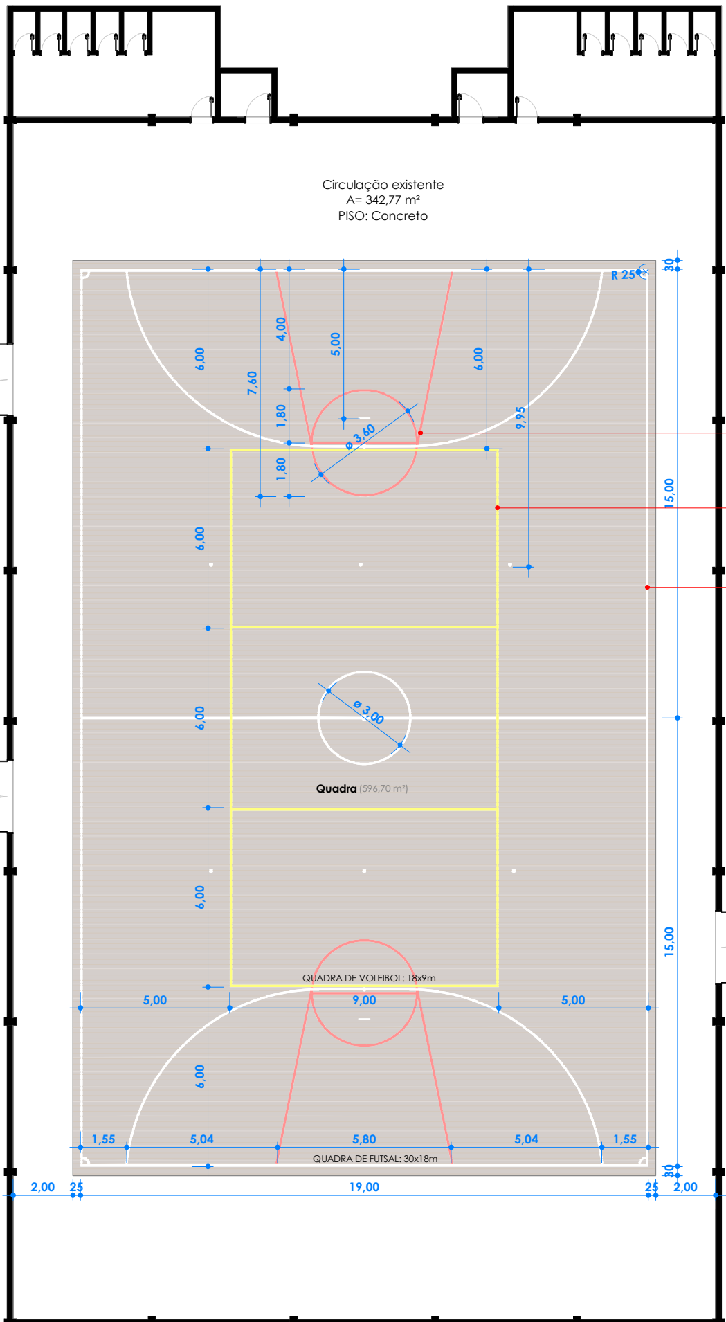
Planta baixa pinturas das linhas | ESCALA: 1 : 175
