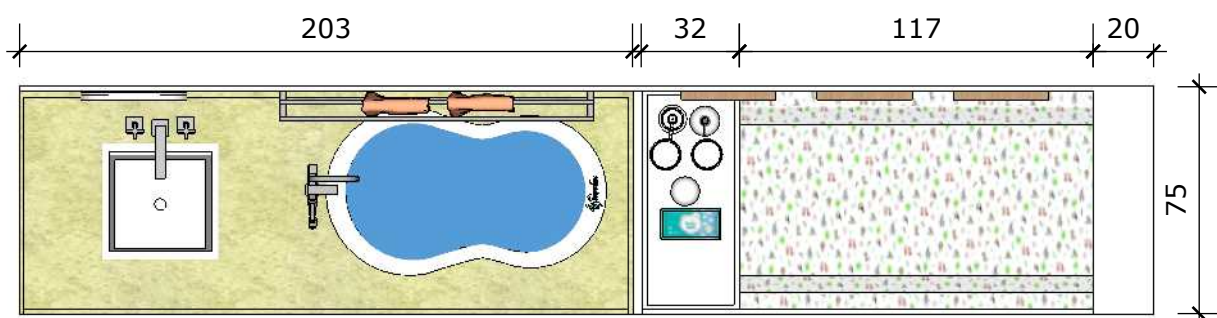
Vista superior Esc.: 1/25
