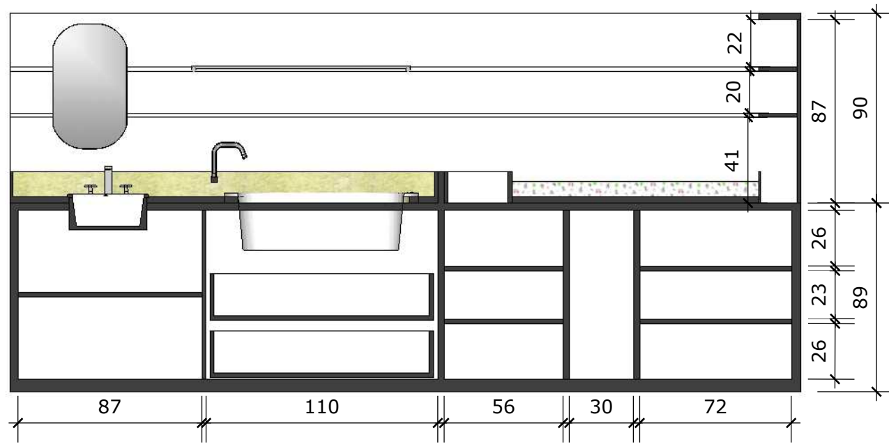
Corte frontal Esc.: 1/25
