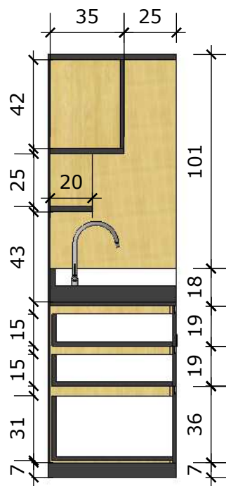
Corte lateral 01 Esc.: 1/25
