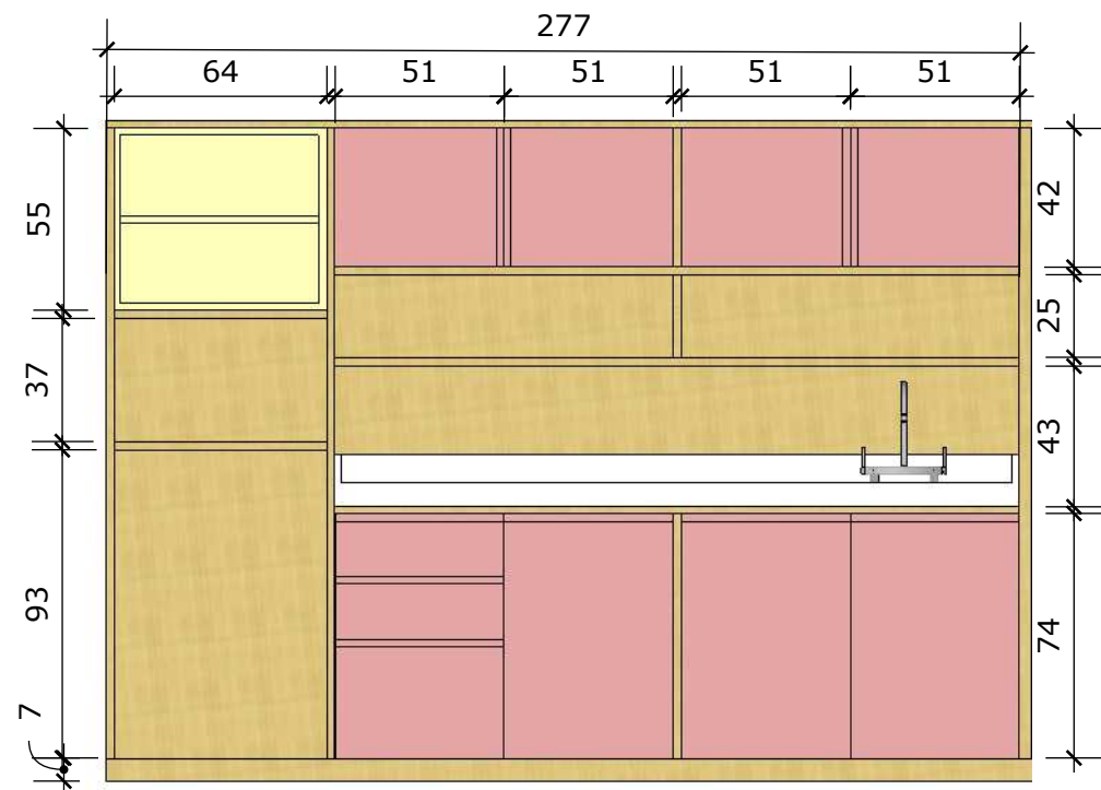
Vista frontal Esc.: 1/25
