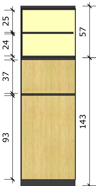
Corte lateral 02 Esc.: 1/25
