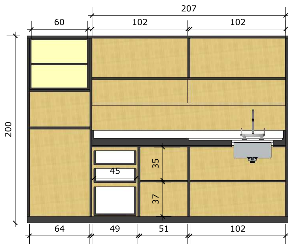
Corte frontal Esc.: 1/25
