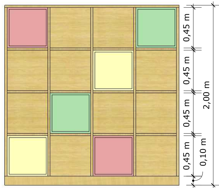
Vista frontal Esc.: 1/25
