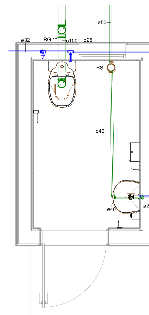
Térreo - Fase 1 - Banheiro PNE ESCALA 1 : 25
