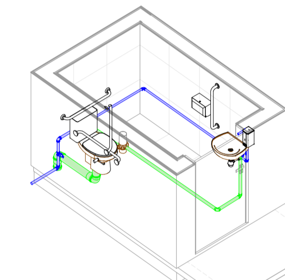
Isométrica - Banheiro PNE ESCALA
