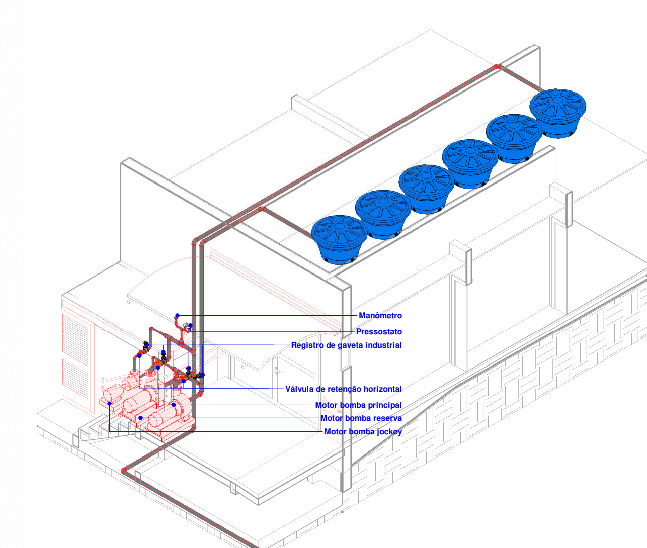
DETALHE BOMBAS ESCALA
