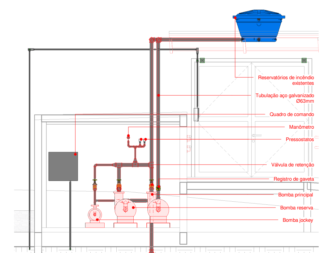
VISTA FRONTAL CASA DE BOMBAS ESCALA 1 : 50
