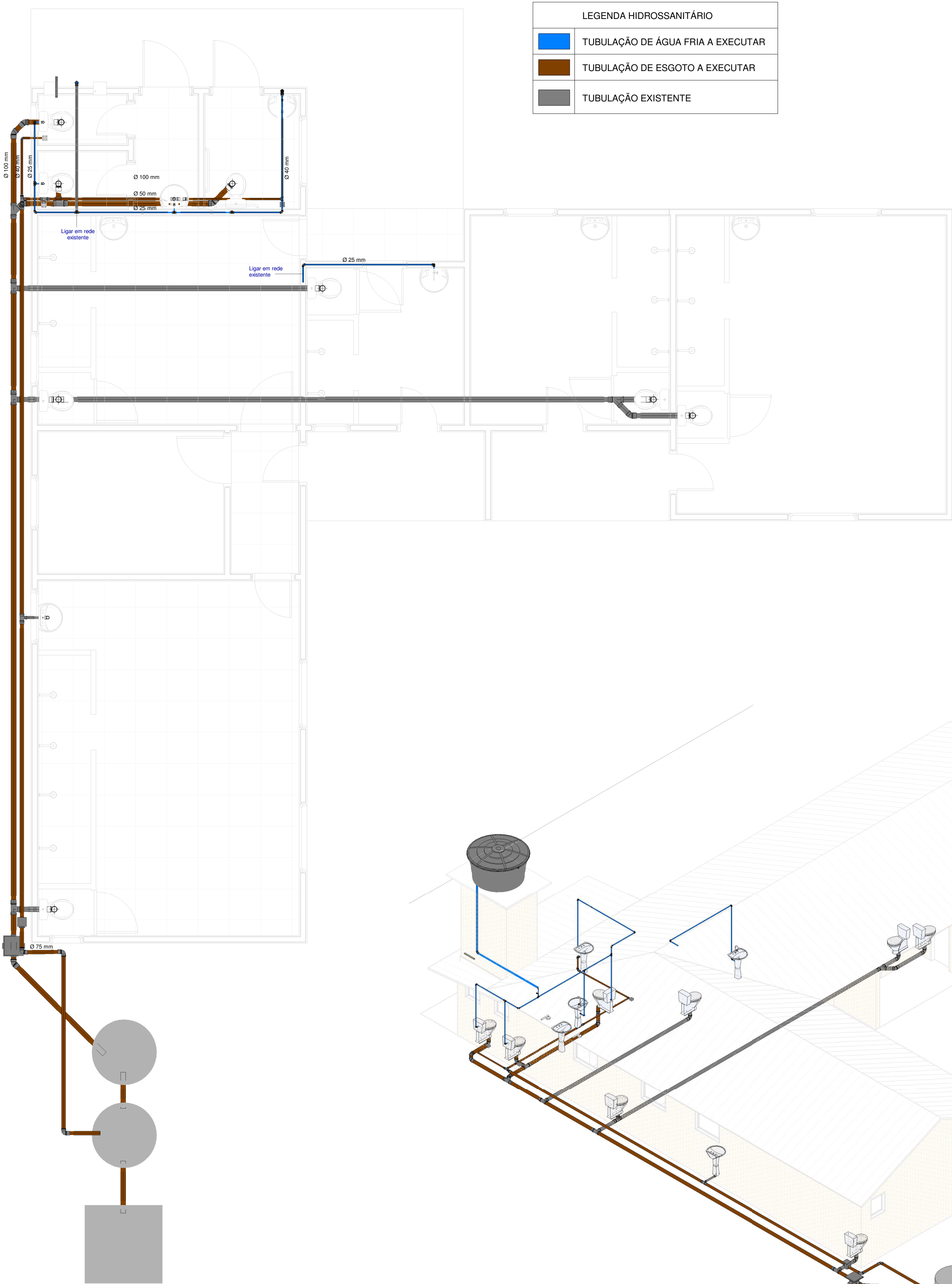
PLANTA HIDROSSANITÁRIA ESCALA 1:50
