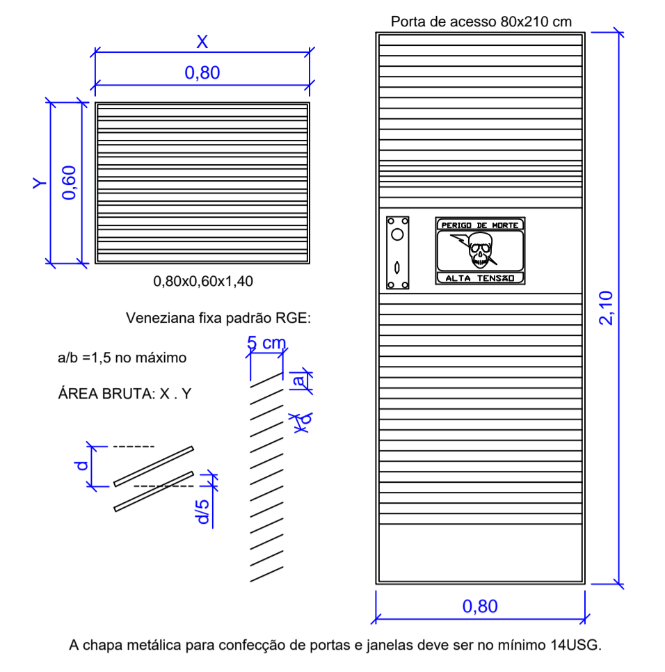
Detalhes aberturas e porta Esc.: 1/20
