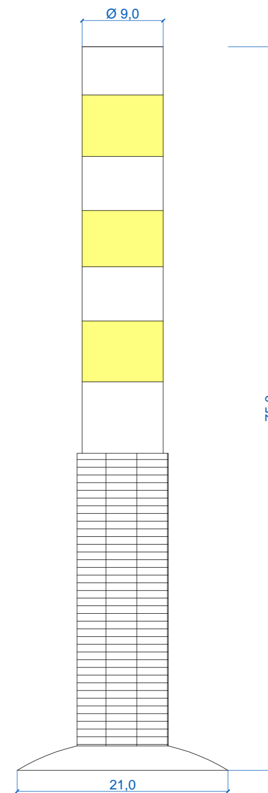
03 Detalhe - Poste Flexível Sem Escala
